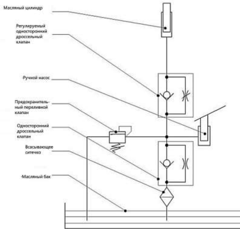
Рис.1 - Схема гидравлической системы
