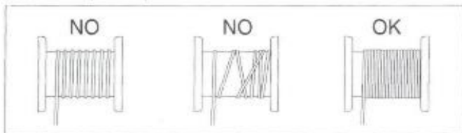
Рис.6 - Намотка троса на катушку
