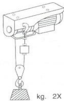
Рис.4 - Установка полиспаста
