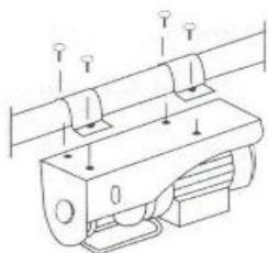
Рис.3 - Установка тали
