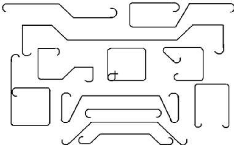
Рис. 2 - Формы изгиба арматуры
